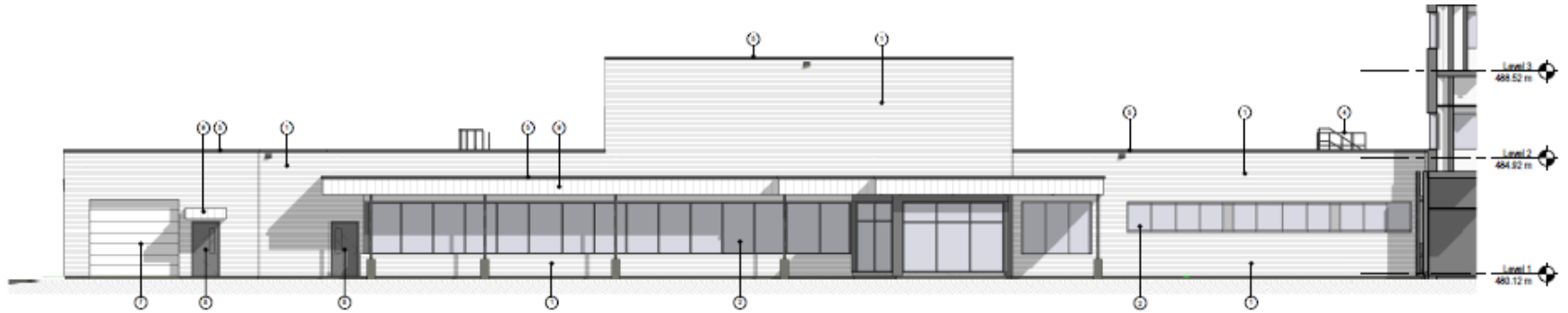
1 WEST ELEVATION A201 1:100
